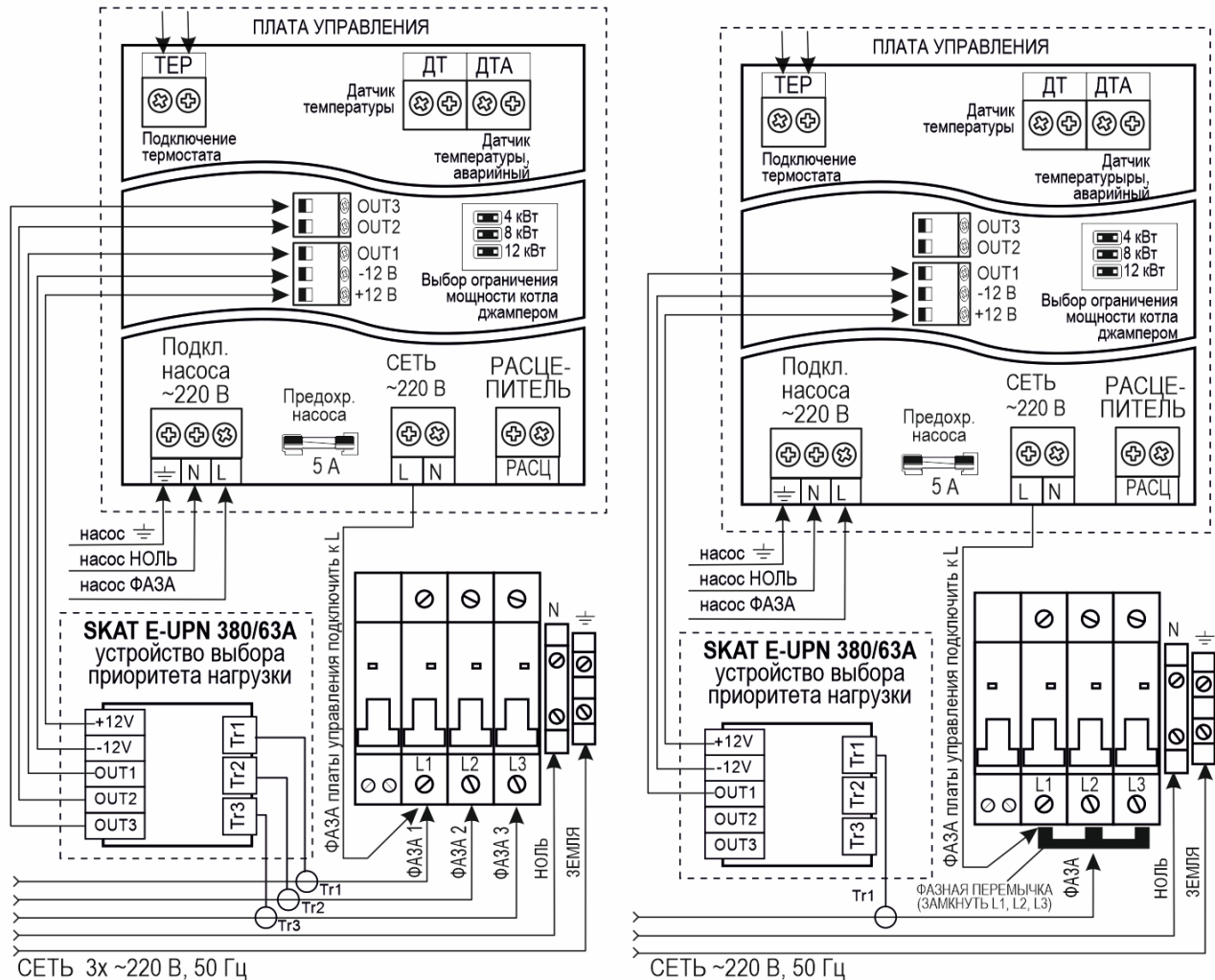
Схема подключения электродкотла к сетям ~220 В и 3х~220 В
